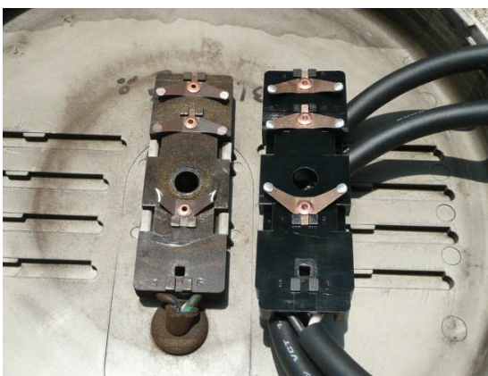
新品との比較及び刃物状に摩耗した1次側接点(左側)
